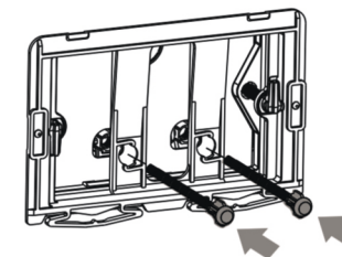
⑨ Установите толкатель.
