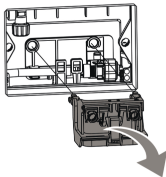
② Выньте подставку для смыва.
