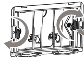
⑧ Установите кронштейн панели, используйте фиксированное соединение «L» для фиксации.
