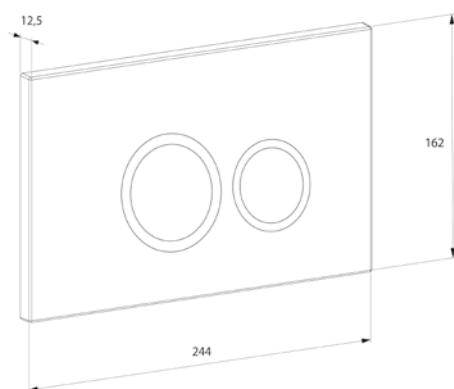
DB1529025 Клавиша смыва D&K Коллекция: Bayern Цвет: черный
